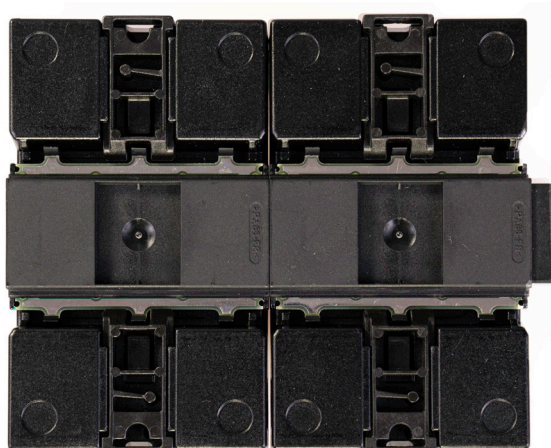
Fig. : Solar-Log Base et MOD I/O assemblés avec connecteur de bus.
