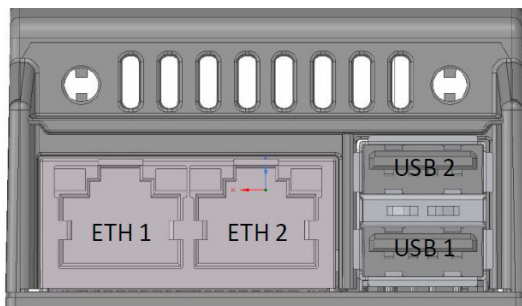
Fig. : Connexions Solar-Log 15 Base – partie inférieure
