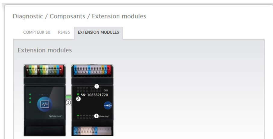
Fig. : Bus de communication/LED Solar-Log MOD I/O - Solar-Log Base
